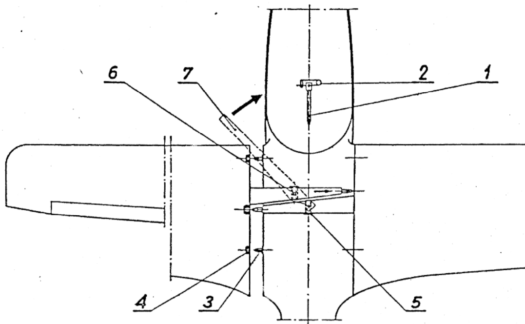
Рис. 6. Монтаж крыла
