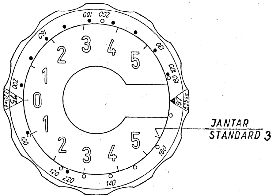
Рис. 5. Расчетный диск планера СЗД-48-3 "ЯНТАРЬ СТАНДАРТ 3" для стандартного исполнения планера
