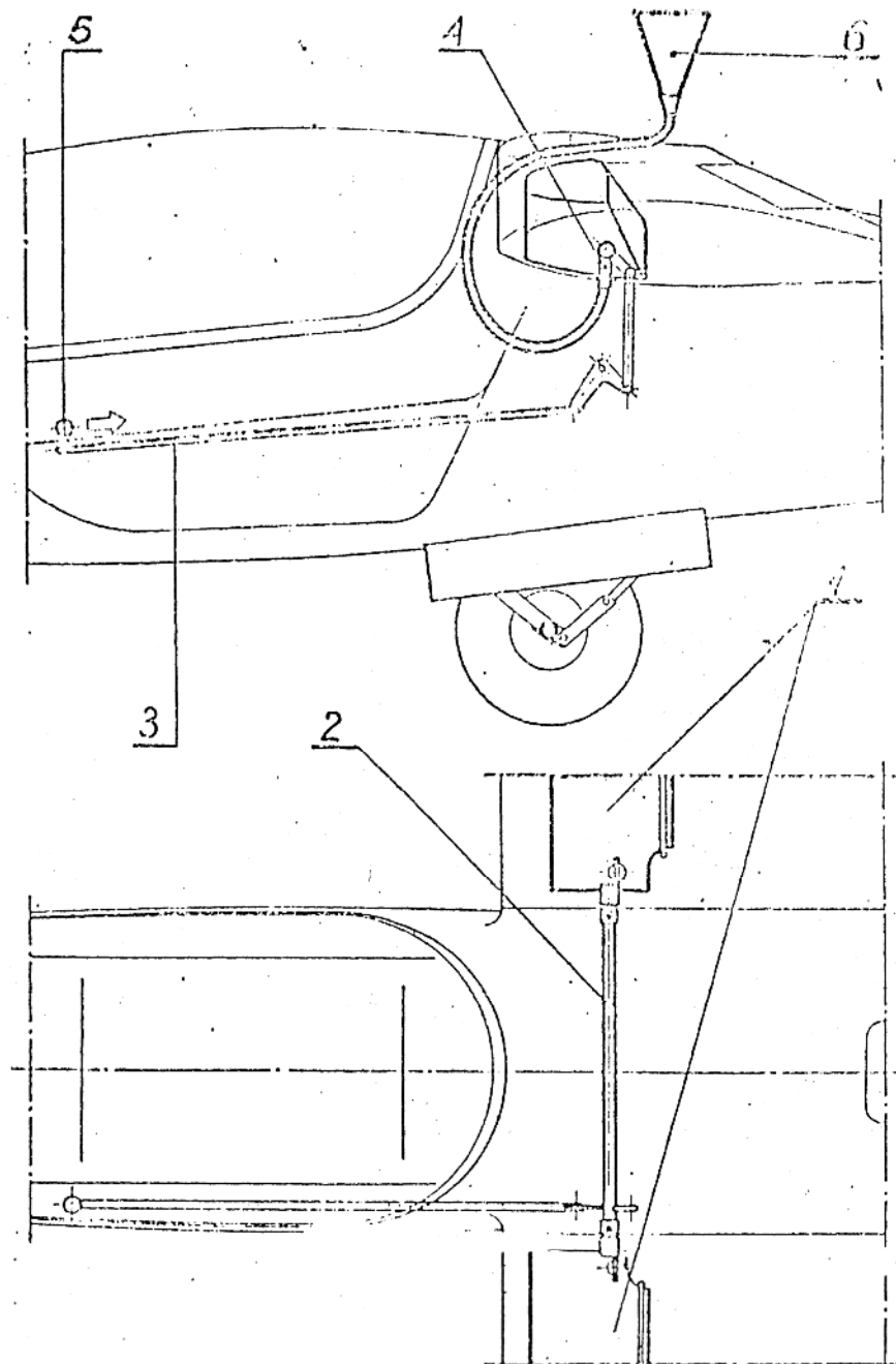
Рис. 3. Система водяного балласта
