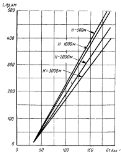
Рис. 2. Дальность полета самолета с колесным шасси в зависимости от запаса топлива при взлете и высоты полета.
