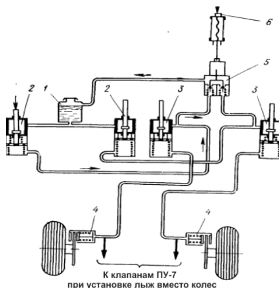
Рис. 7. Схема гидросистемы
